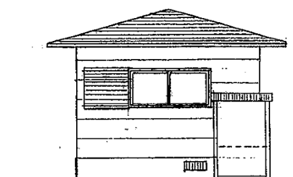
東立面図
