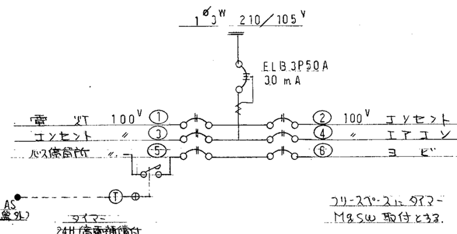
分電盤 結線図
