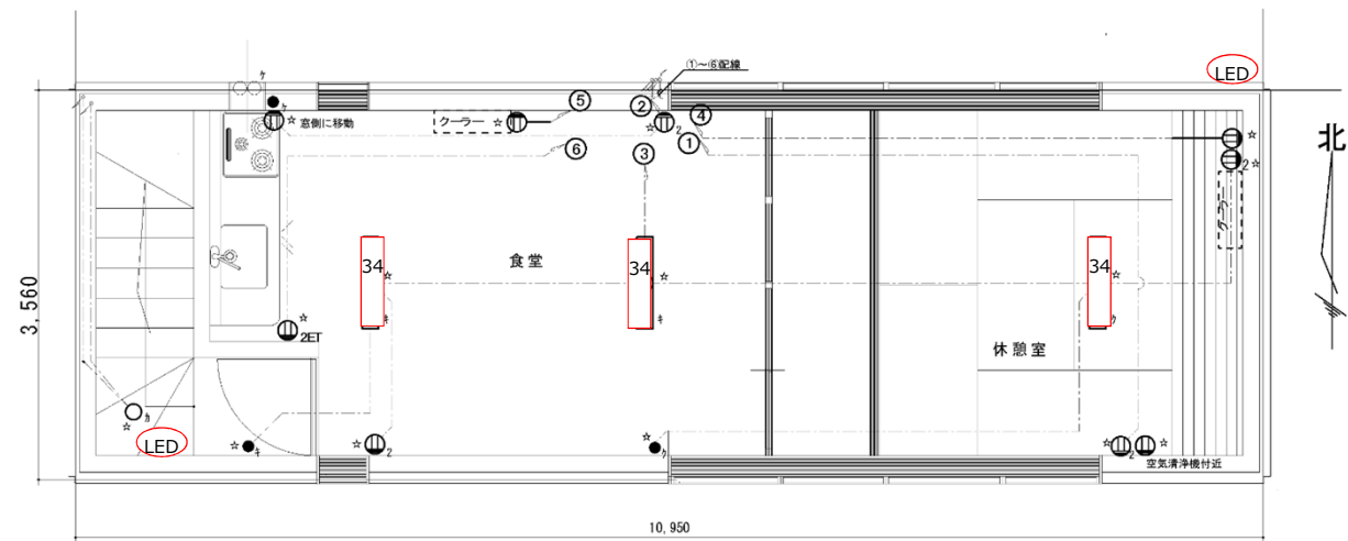
2 階平面図
