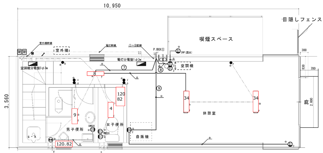
1 階平面図
