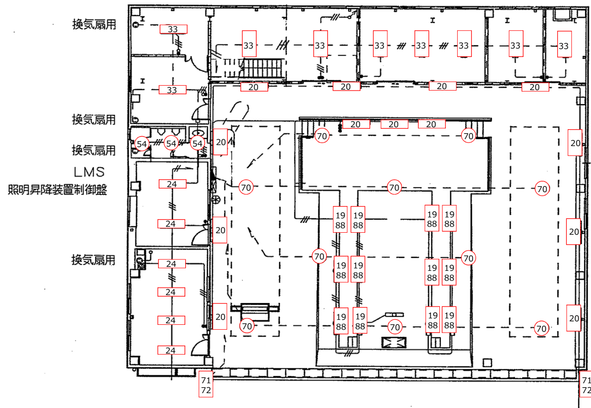
整備工場 1 階
