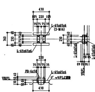
照明受付架台詳細図 S=1/30
